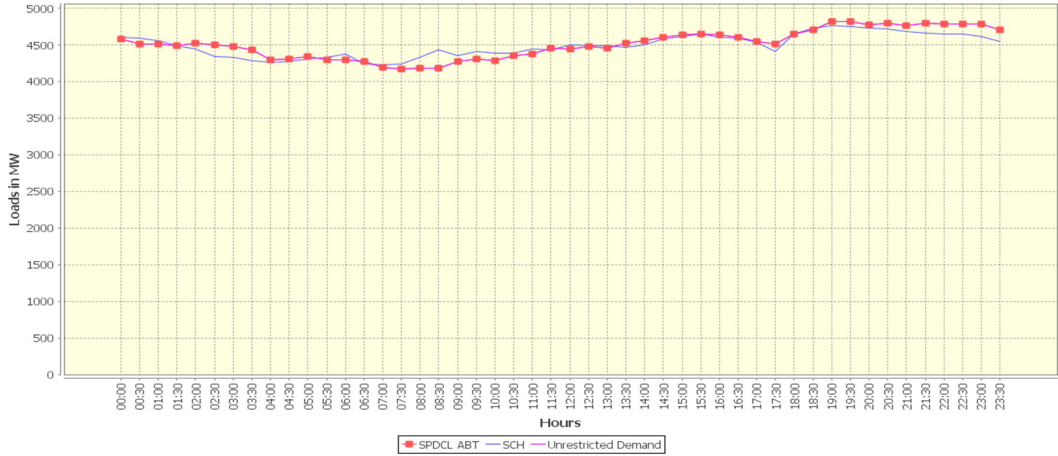
TSSPDCL-LMRC/Corporate Office SPDCL Load Vs Schedule for 20.05.2018 ( Sunday )
